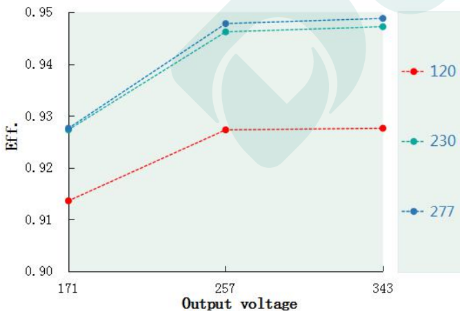
Eff. VS Output voltage(DL-240W-V343A/P/X-MXG)
