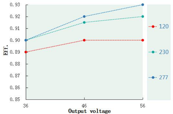
Eff. VS Output voltage(DL-240W-V56A/P/X-MXG)
