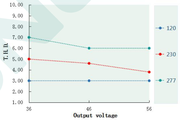
T.H.D. VS Output voltage(DL-240W-V56A/P/X-MXG)
