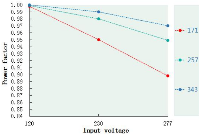
Power factor VS Input voltage(DL-240W-V343A/P/X-MXG)
