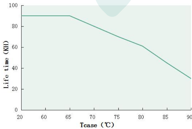
Tcase VS Lifetime(DL-240W-A/P/X-MXG)
